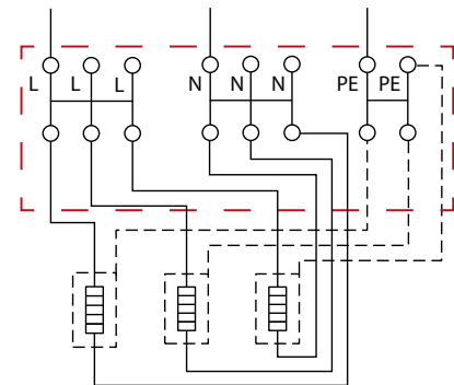
Соединение трех ELSR нагревательных кабелей
