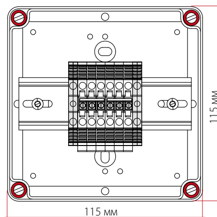
Соединение трех ELSR нагревательных кабелей
