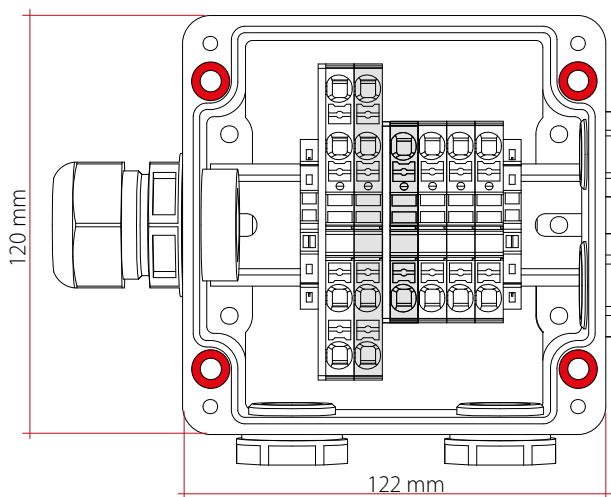
Sternpunkt ELK-MI-Twin & Sternpunkt 3-Phasen ELK-MI-Single
