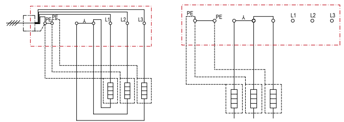
Sternpunkt ELK-MI-Twin & Sternpunkt 3-Phasen ELK-MI-Single
