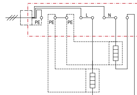
In Reihe geschaltet mit Spleißkit
