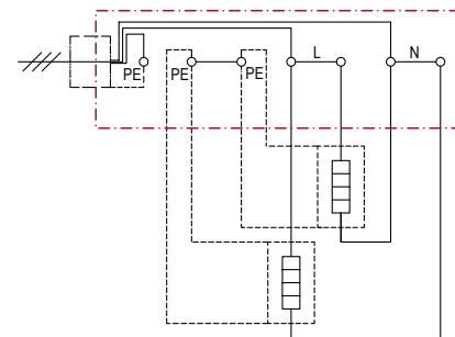
Parallel geschaltet
