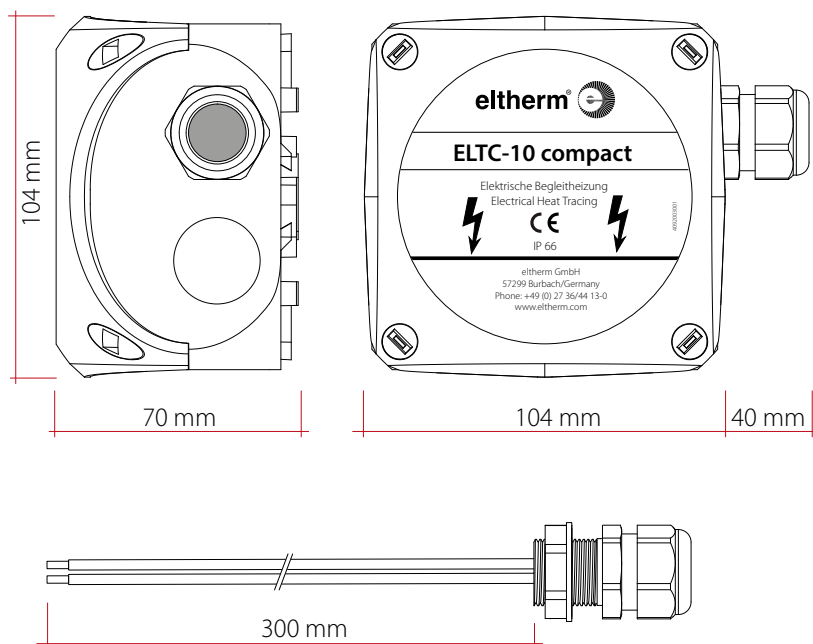
Abmessungen
