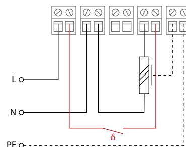
Schaltbild
