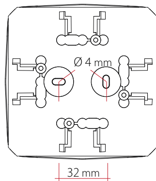
Bohrbild
