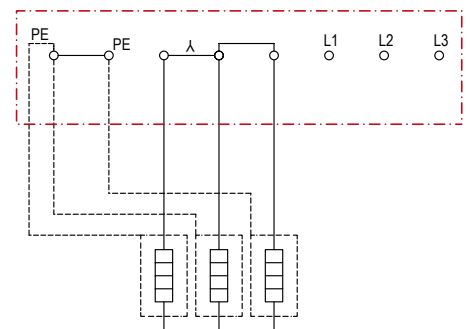
Sternpunkt 3-Phasen ELK-MI-Single
