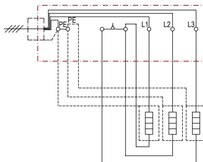
Anschluss & Sternpunkt ELK-MI-Twin
