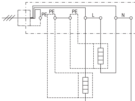
Parallel geschaltet
