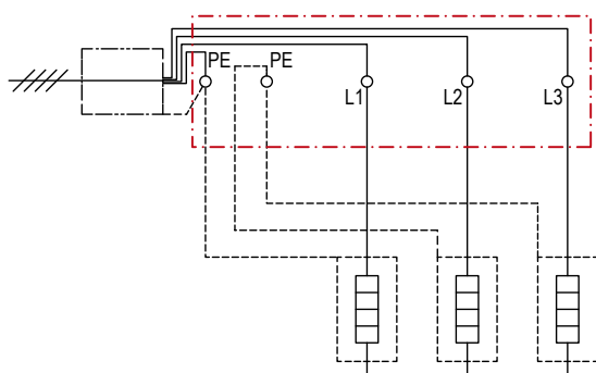
3 Phasen geschaltet
